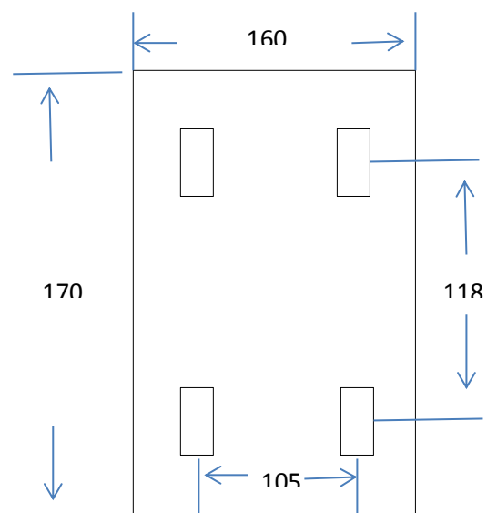
Mått motorns bottenplatta
